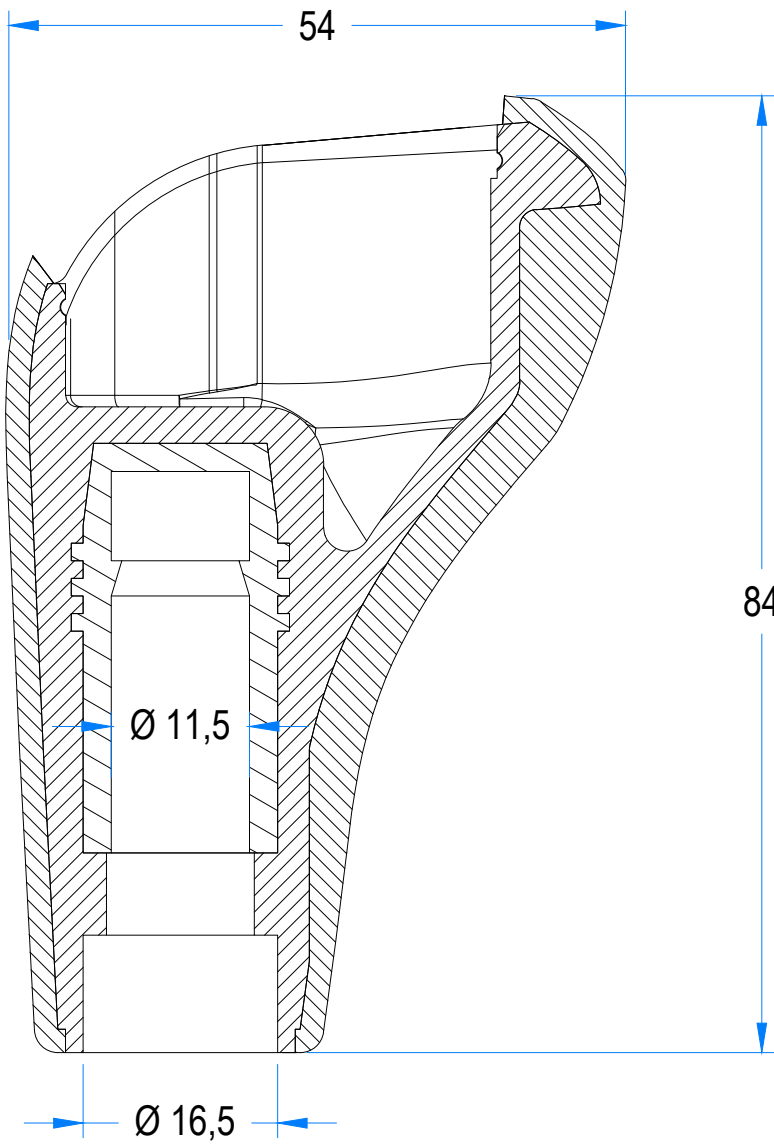
A-A Section
