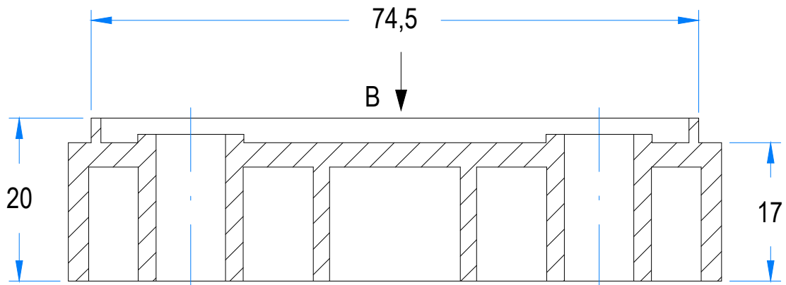
A-A Section
