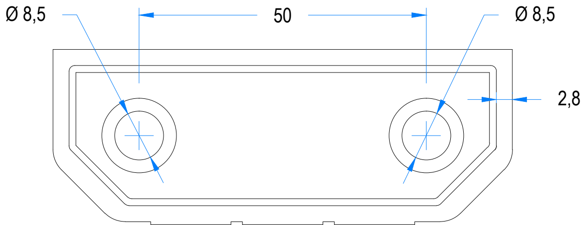
B Wiew
